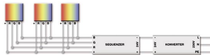
Schaltplan / wiring diagram
